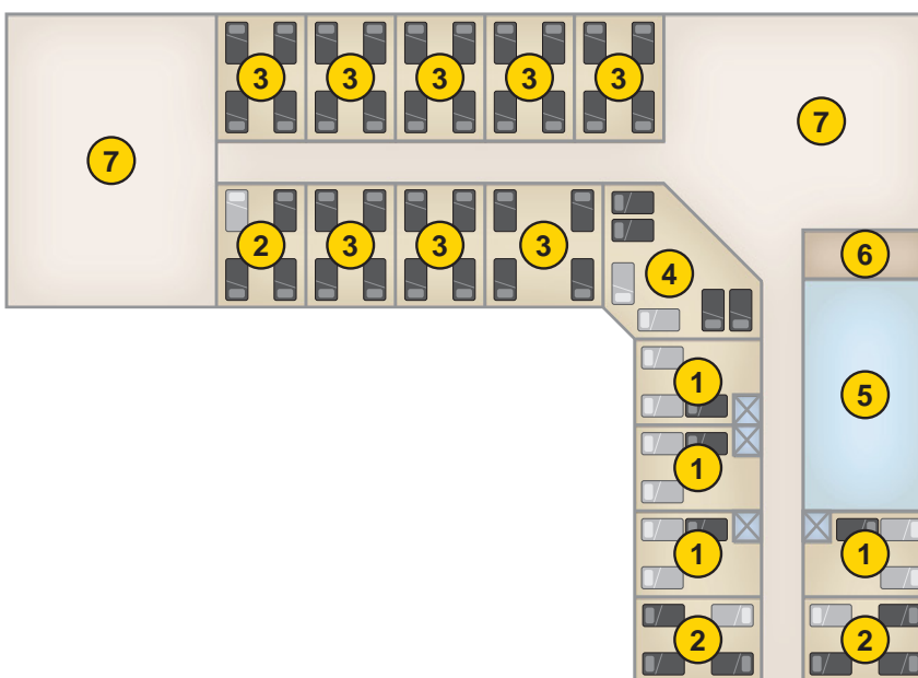
ALAPRAJZ EMELET
